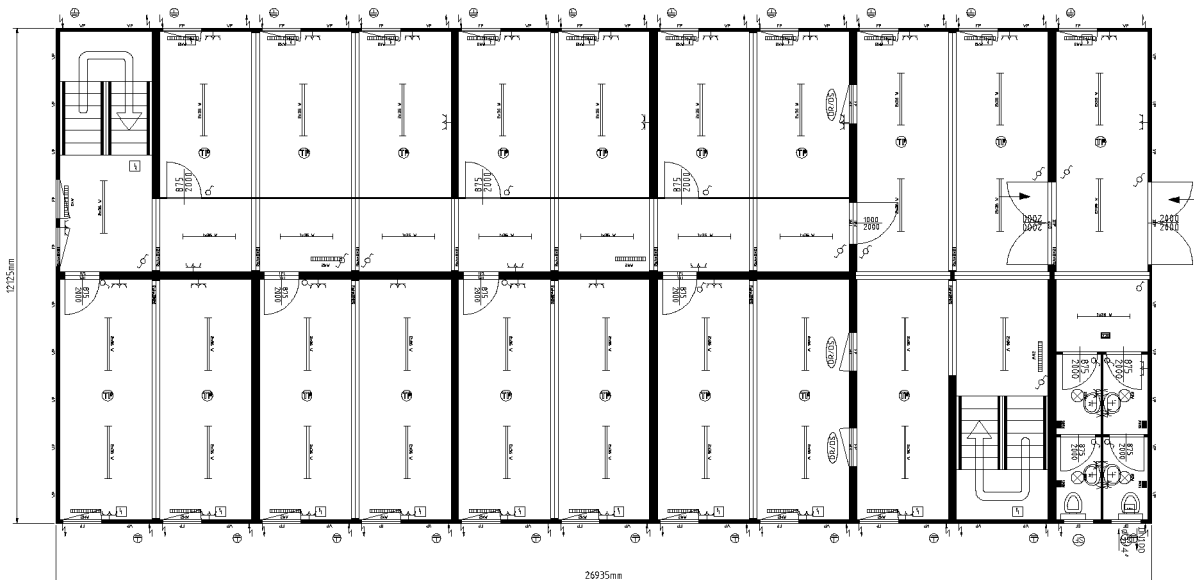
первый этаж
